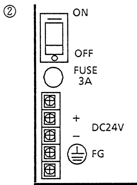
本体裏面図
