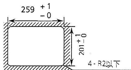
① 取り付け穴詳細図 (単位:mm)
