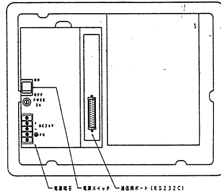
裏面図
