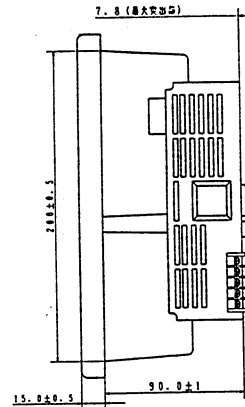
側面図
