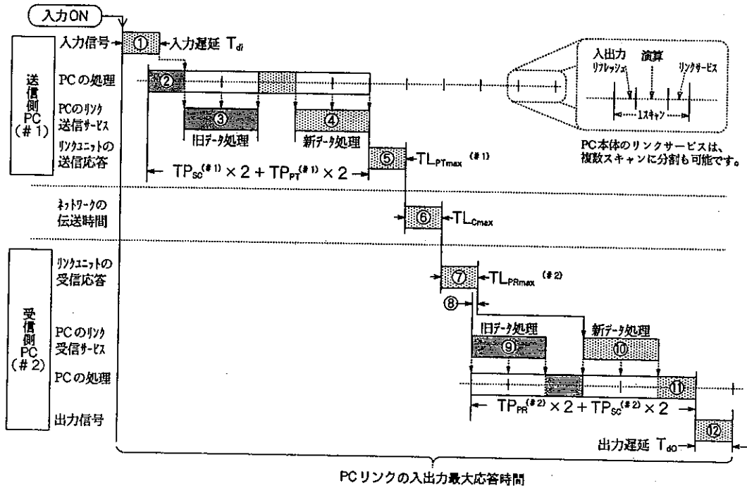
伝送応答時間が最大になる場合のタイムチャート
