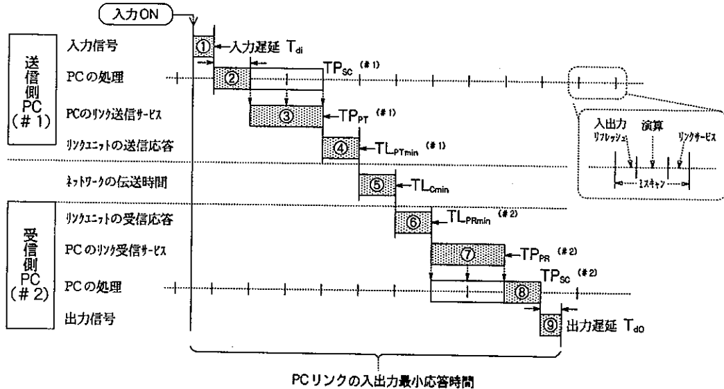
伝送応答時間が最小になる場合のタイムチャート
