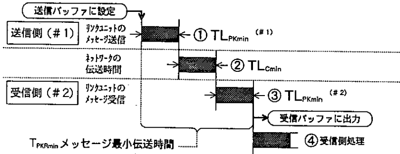
伝送時間が最小になる場合のタイムチャート
