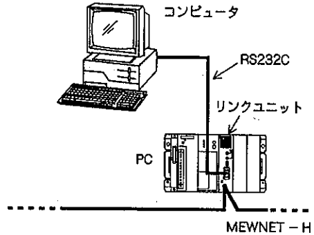
上図はリンクユニットのRS232Cインターフェースに接続した例です
