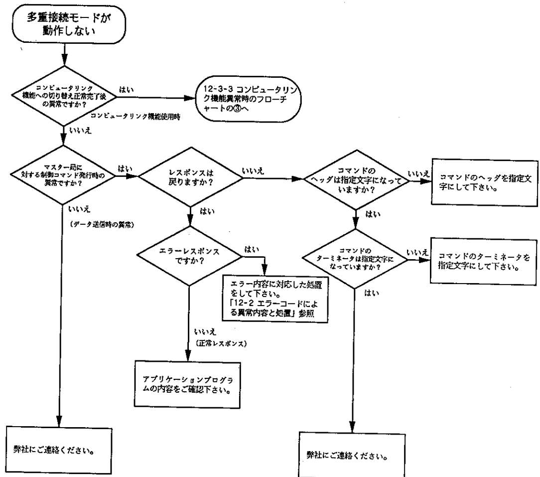
a. 多重接続モード異常時のフローチャート
