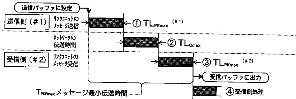
伝送時間が最大になる場合のタイムチャート
