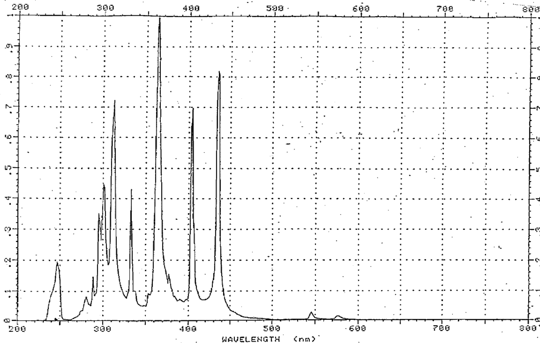
パナキュアー スポットタイプ ANUP5252L-分光分布特性 (ANUPS252)
