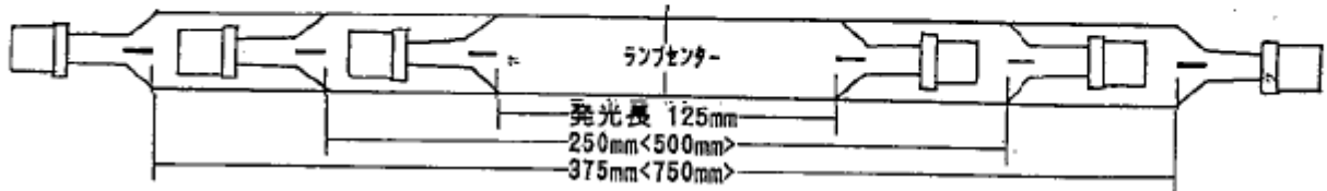
UVランプ 平行方向強度データ (参考値)
